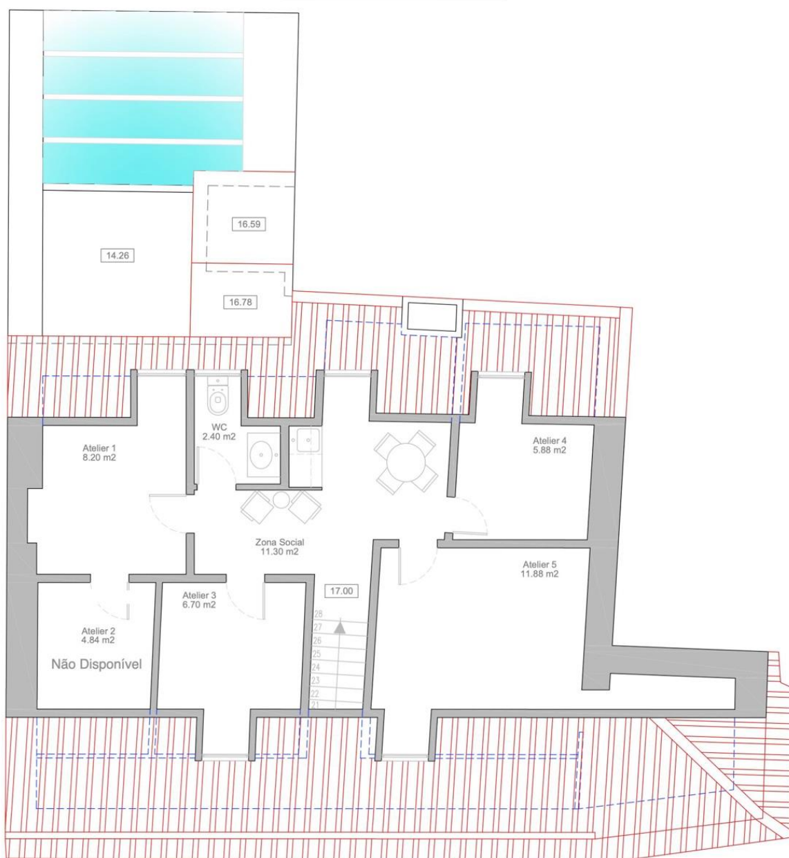
PLANTA DO SOTÃO SOLUÇÃO-C-ESC: 1/50
